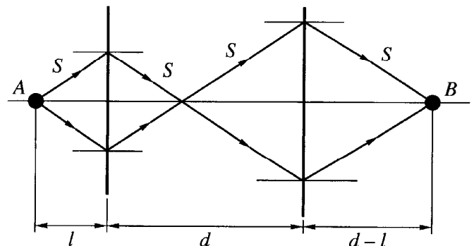
Рис. 2. Ход лучей ( S ) в линзе Веселаго, A – источник, B – изображение источника, d – толщина пластины, L – расстояние от источника до пластины
