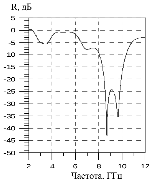
Рис. 10. Частотная зависимость коэффициента отражения образца композита, состоящего из комбинированных спиралей различных диаметров
