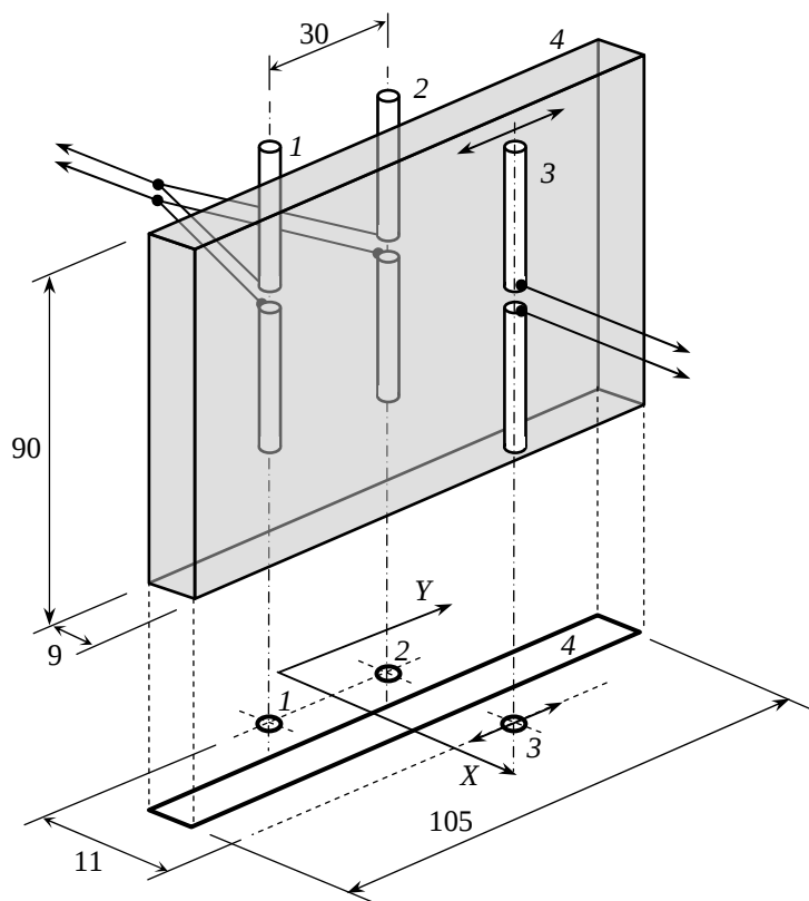
Рис. 15. Схема эксперимента
