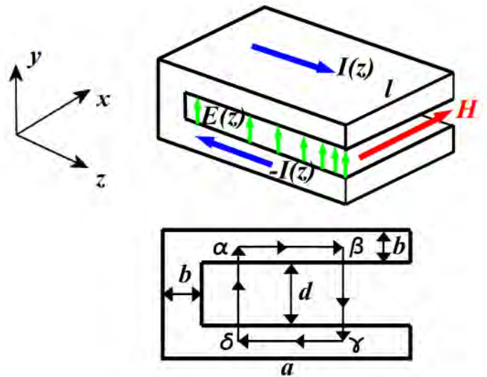
Рис. 18. Нано-антенна в виде подковы (наноподкова); при компьютерном моделировании использовались параметры a = 300 нм, d = 70 нм, b = 34 нм
