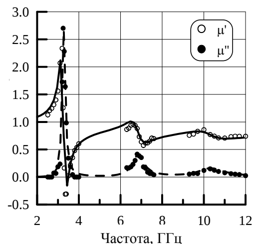
Рис. 5. Эффективная магнитная проницаемость композита с сегнетокерамическими включениями кубической формы
